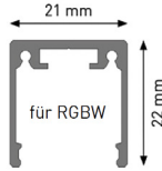
Clip 22
